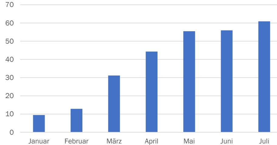
PV-Stromerzeugung [MWh]
